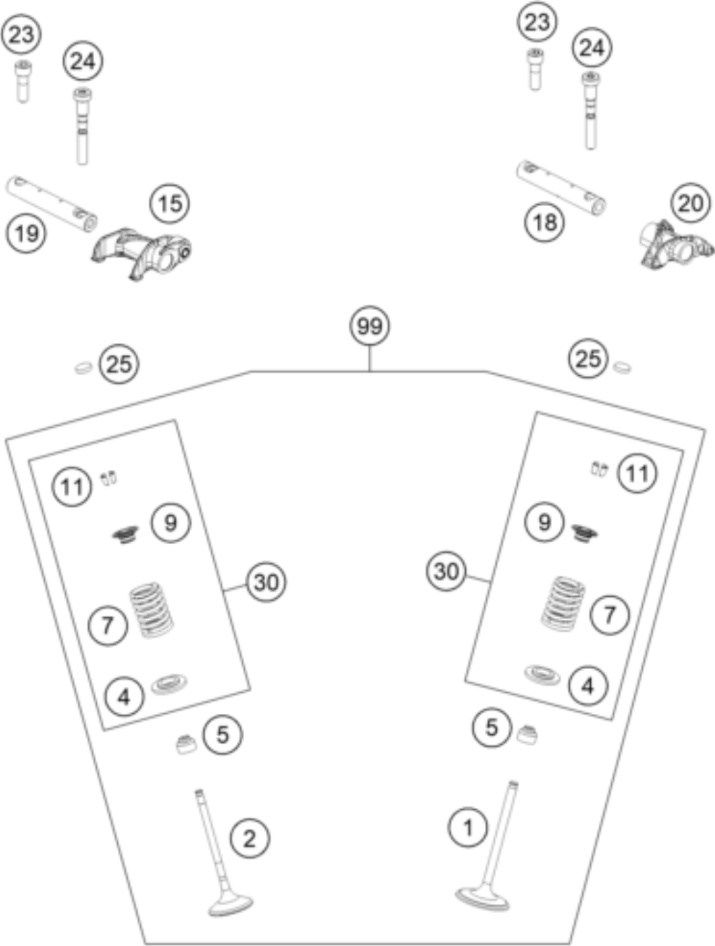
AUSLASS / EXHAUST
